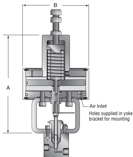
Air-to-Open (ATO)
