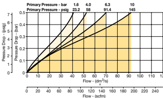
P33LA 1/2" Lubricator
